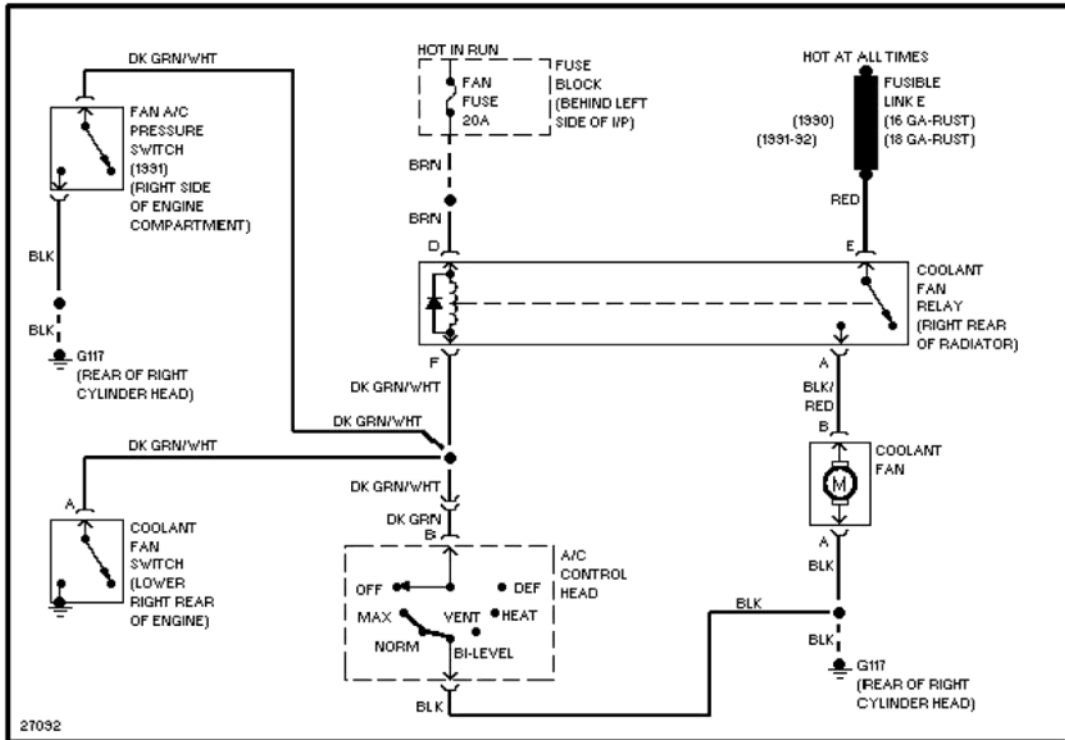
5.0L (VIN E), Cooling Fan Circuit
