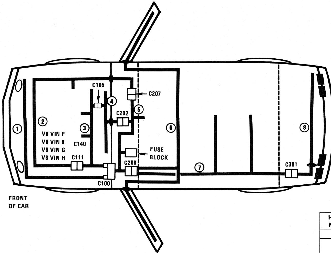
HARNESS CHART (V8 VIN F, V8 VIN 8, V8 VIN G, V8 VIN H)
