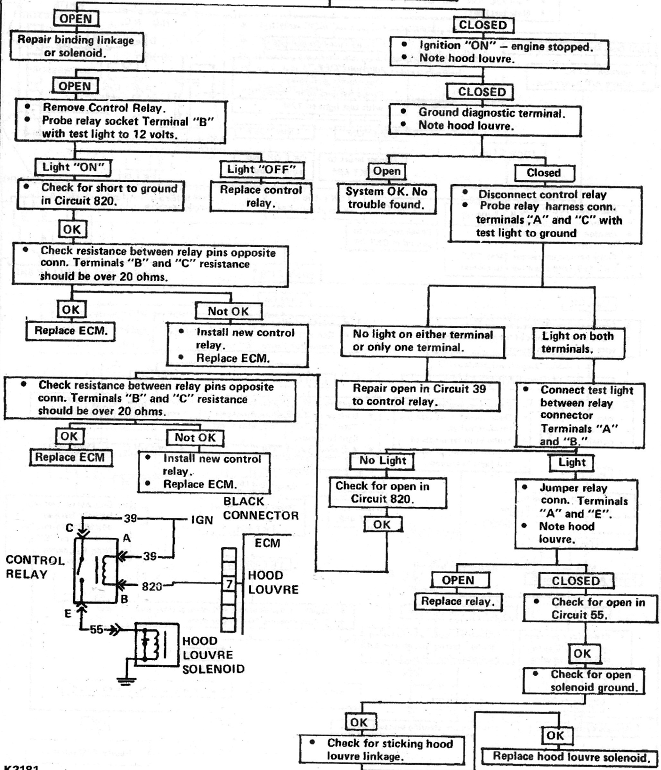
Fig. 6E2-46 Hood Louvre Solenoid-5.0L
